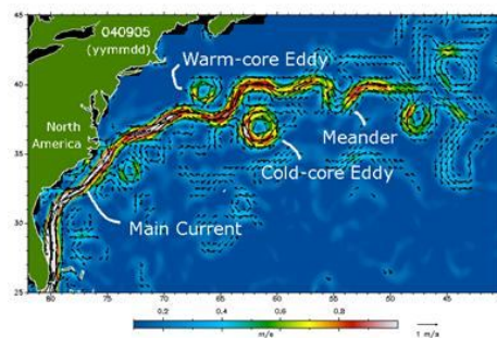
Snelheden in een normale Warme Golfstroom, september 2004
