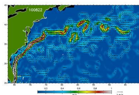
Warme Golfstroom snelheden 15 augustus 2010
